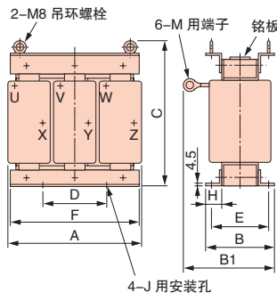
外形图2
