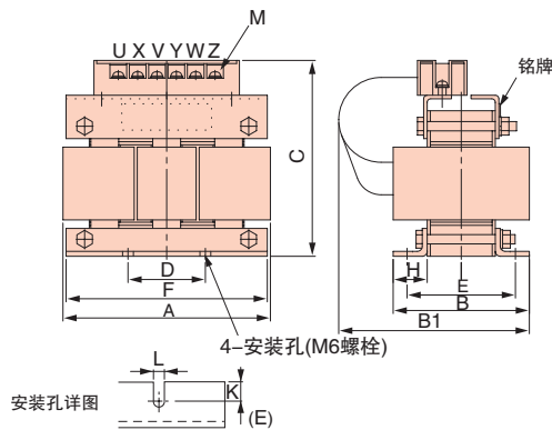
外形图2
