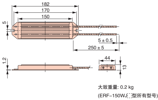
ERF-150WJ系列
