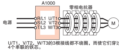
接线图b
