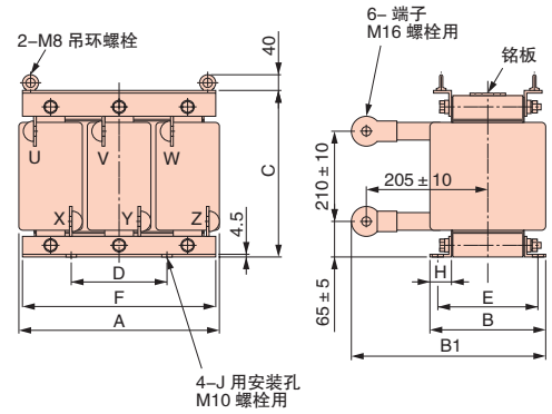
外形图3
