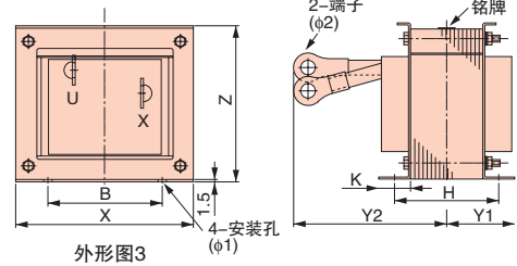
外形图3
