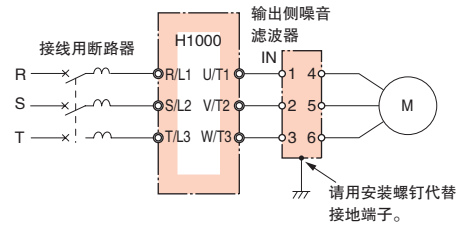
接线图
