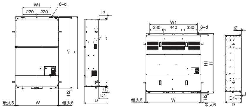
外形图3
