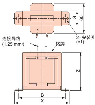
外形图1
