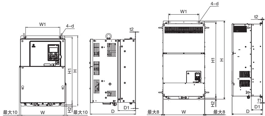
外形图1
