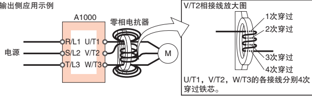
接线图a
