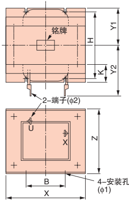
外形图2
